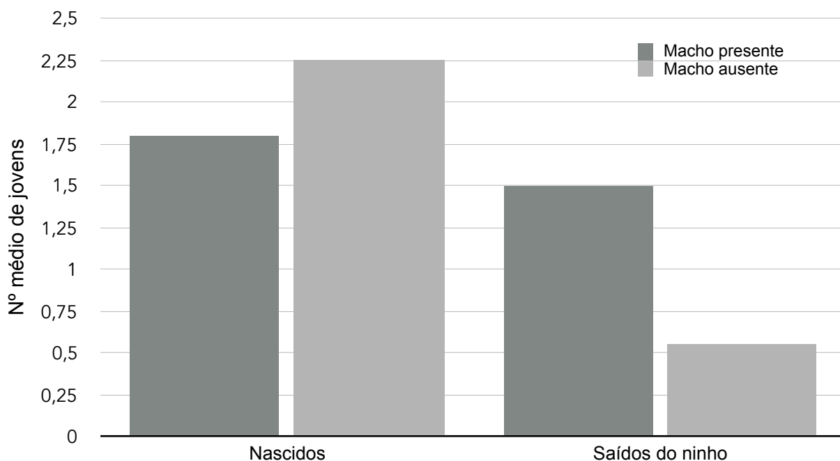
Figura 1. Números de nascimentos de pintos com diferentes sistemas de acasalamento.
